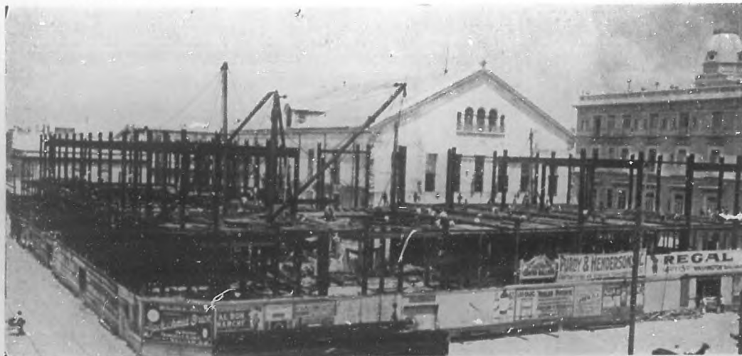
Vista de la armazón de acero, fabricada en los talleres de esta Compañía, del edificio del Centro Gallego, en sus comienzos. TALLERES Y ALMACENES EN HACENDADOS DE 12.000 TONELADAS DE CAPACIDAD. OFICINA: EMPEDRADO NUM. 17, HABANA
